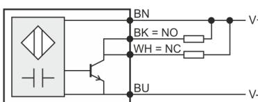
(i)DOL 26 NPN
