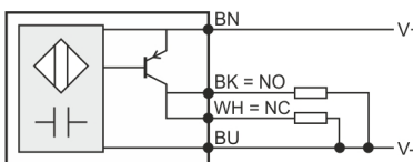
(i)DOL 26 PNP
